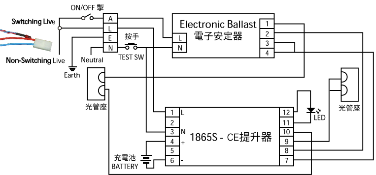
1865S 電子安定器的接線圖 (長明式/後備式)
